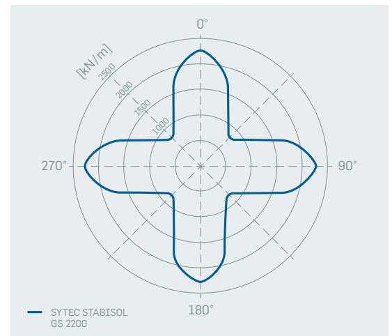
Rigidità all'allungamento radiale
